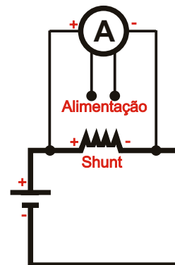
Amperímetro Digital (CC) ligado a Shunt
