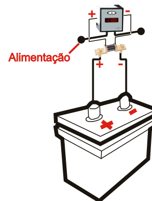
Amperímetro Digital (CC) ligado a Shunt
