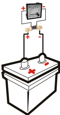
Amperímetro (CC) ligado a Shunt
