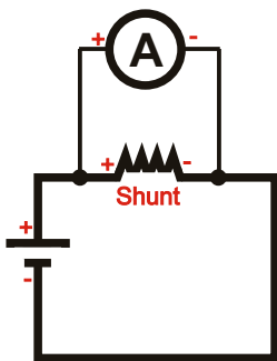
Amperímetro (CC) ligado a Shunt
