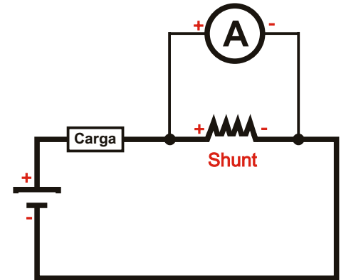
Amperímetro (CC) ligado a Shunt
