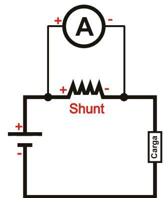
Amperímetro (CC) ligado a Shunt
