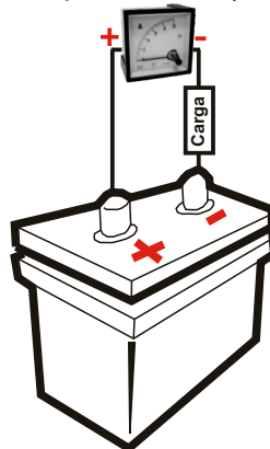
Amperímetro (DC)
