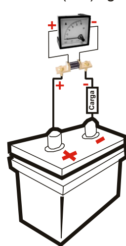
Amperímetro (DC) ligado a Shunt
