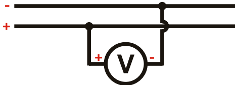
Voltímetro (DC)
