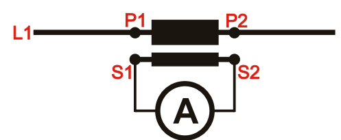
Amperímetro (AC) ligado a TC
