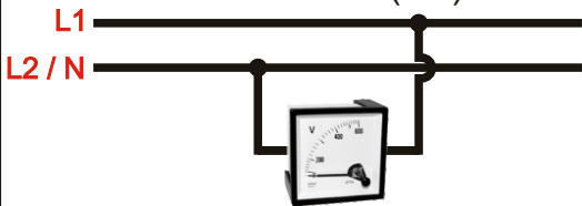
Voltímetro (AC)
