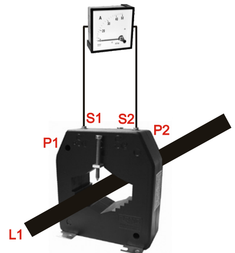
Amperímetro (AC) ligado a TC
